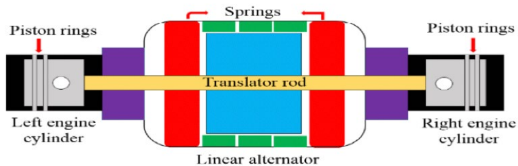
Fig. 24 Vrije zuigermotor [5]
