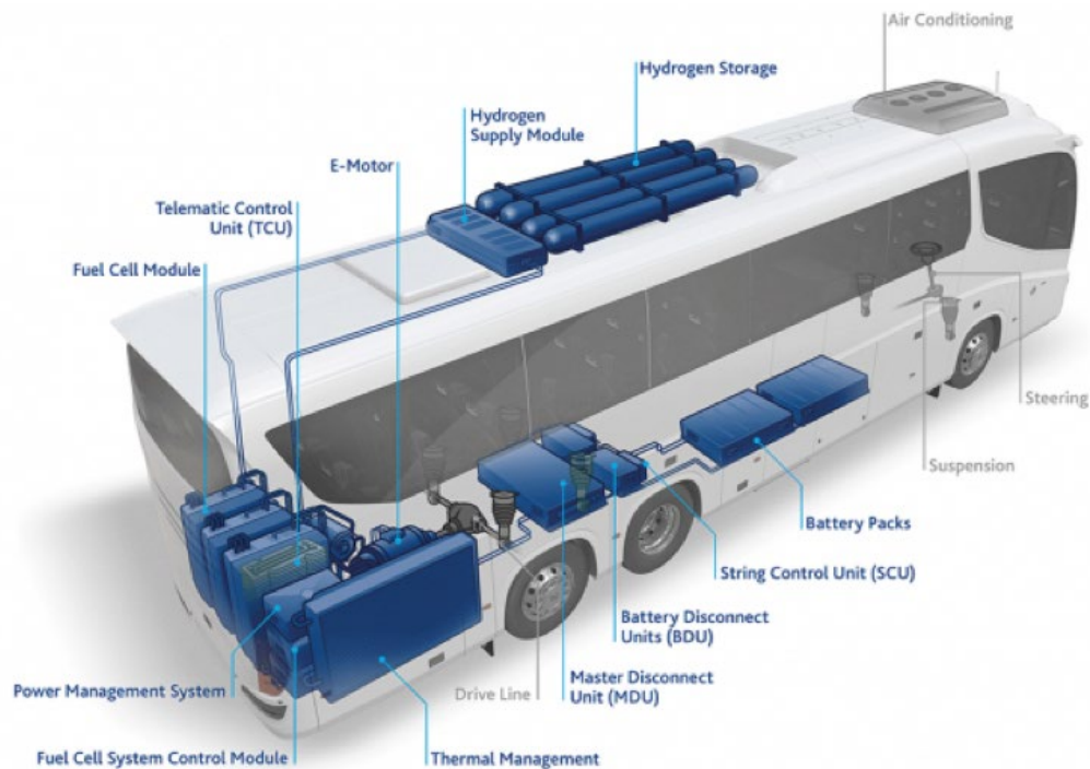
Fig. 21 Compleet brandstofcelsysteem [2]
